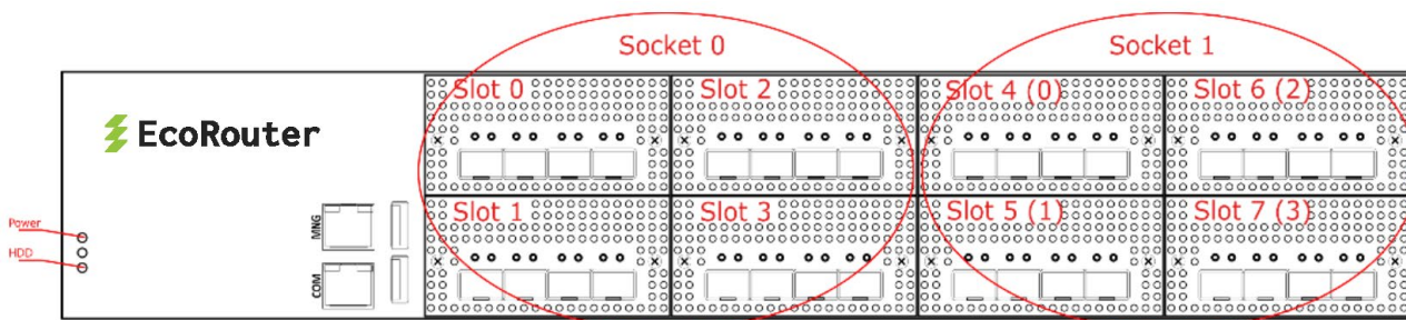
Рисунок 3. Передняя панель ER-2008.
