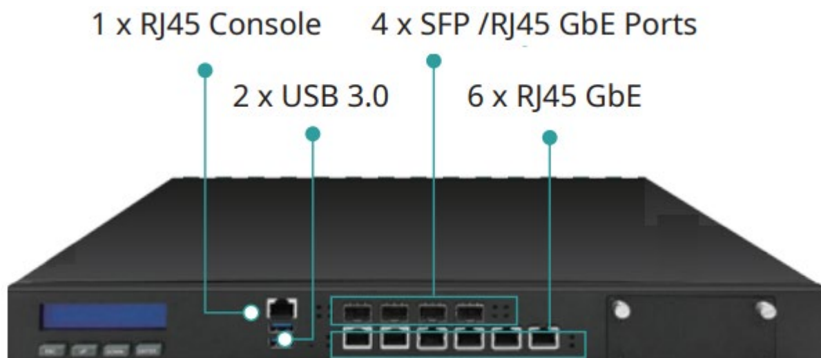
Рисунок 1 Передняя панель ER406
